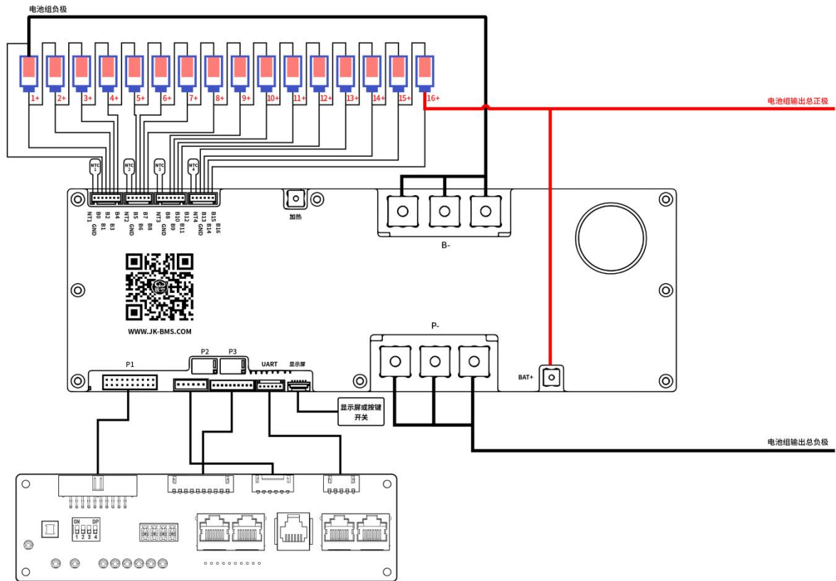
JK-PB2A16S-30P 接线图
