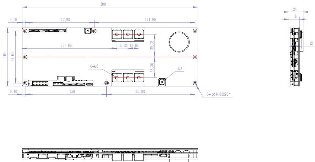
JK-PB2A16S-30P 外形尺寸
